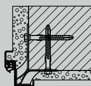
Монтаж при помощи дюбельных анкеров
