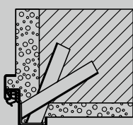
Монтаж при помощи анкеров для кирпичной кладки
